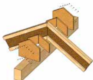
Schéma skladby přílozek
