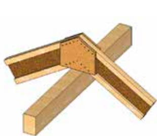
Konstrukce krokví s vrcholovou vaznicí
